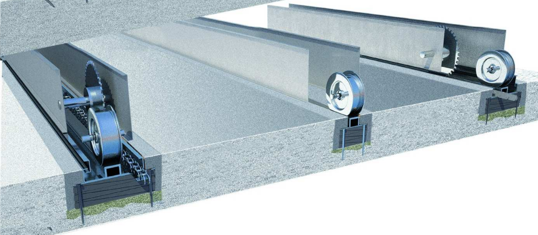
Raíles empotrados
