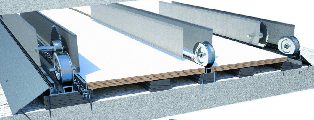
Raíles con suelo melaminado
